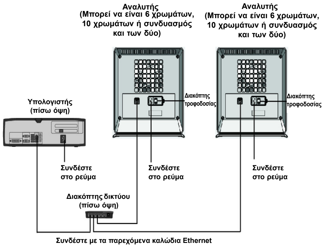
Εικόνα 2-9. Σύνδεση πολλαπλών αναλυτών GX-IV σε σταθερό υπολογιστή
