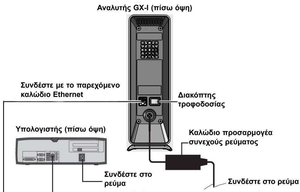
Εικόνα 2-1. Σύνδεση του αναλυτή GX-I σε σταθερό υπολογιστή
