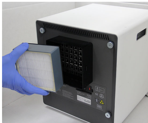
9-28. ábra A HE-szűrő eltávolítása
