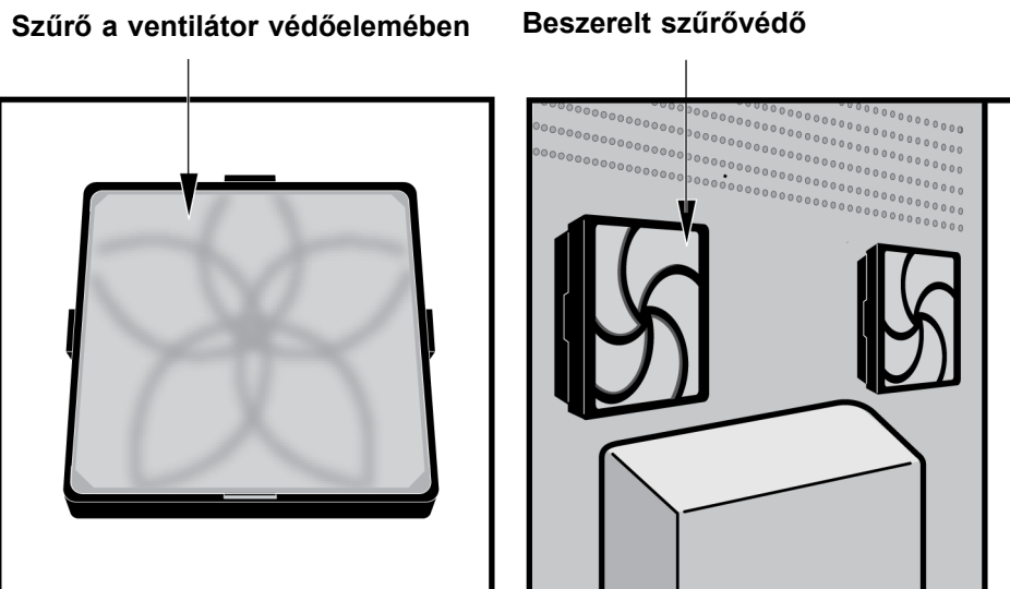
9-20. ábra Csereszűrő és védőelem felszerelve
